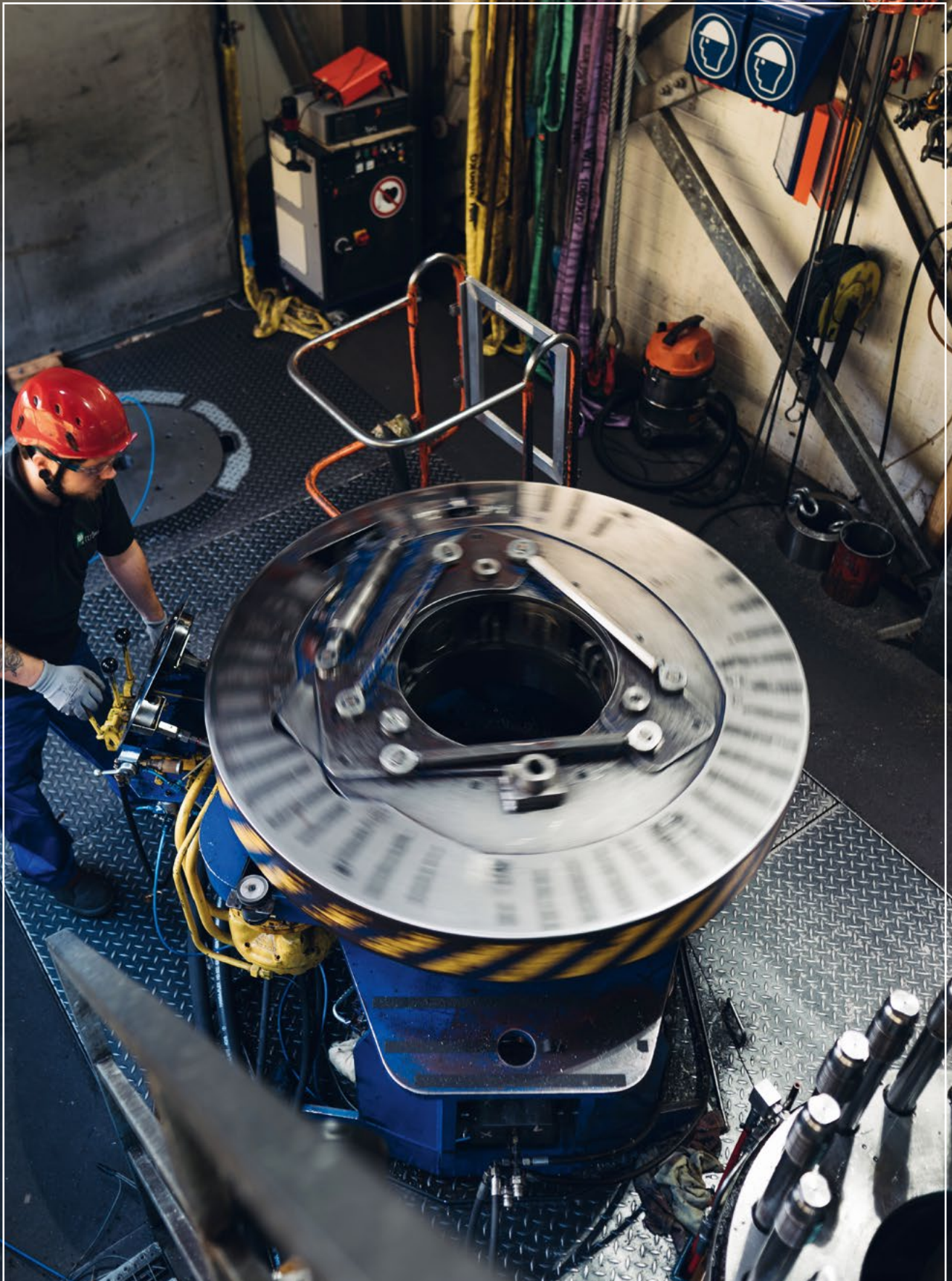
Der geologische Untergrund bietet vielfältige Potenziale für die Speicherung großer Gasvolumina. Das Institute of Subsurface Energy Systems beschäftigt sich mit der Injektion in poröse Medien und Gesteine.
